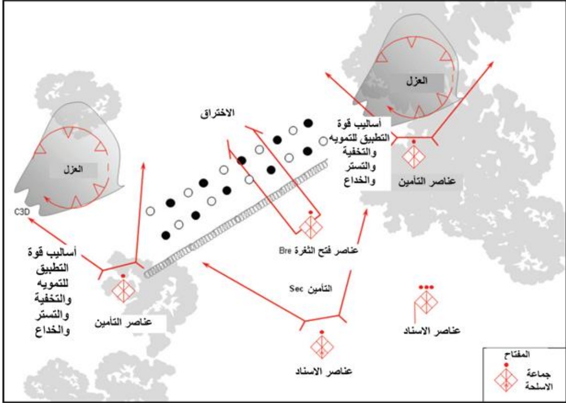
الشكل رقم (24) مثال على فتح الثغرة
